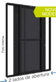
PBCV 3FM Porta Balcão de Correr Veneziana - 3 Folhas Móveis 216X160X9,4 - 3 • 78.50.702-0 Vidro temp. abaixo de 1,10m de altura
