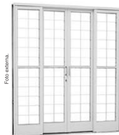
PCQ 4F Porta de Correr com Grade Quadrículada - 4 folhas 217x200x12 - 4 • 26.32.450-5 Vidro Temperado abaixo de 1,10m de altura.*
